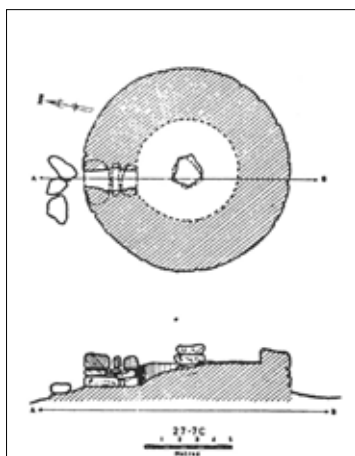
20. Planta i alçat del talaiot de sa Casa Nova de Pina.
